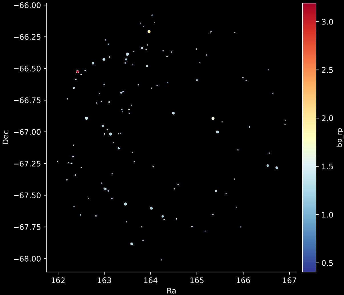
GALAH DR4 Field: [7209] Stars: 119
