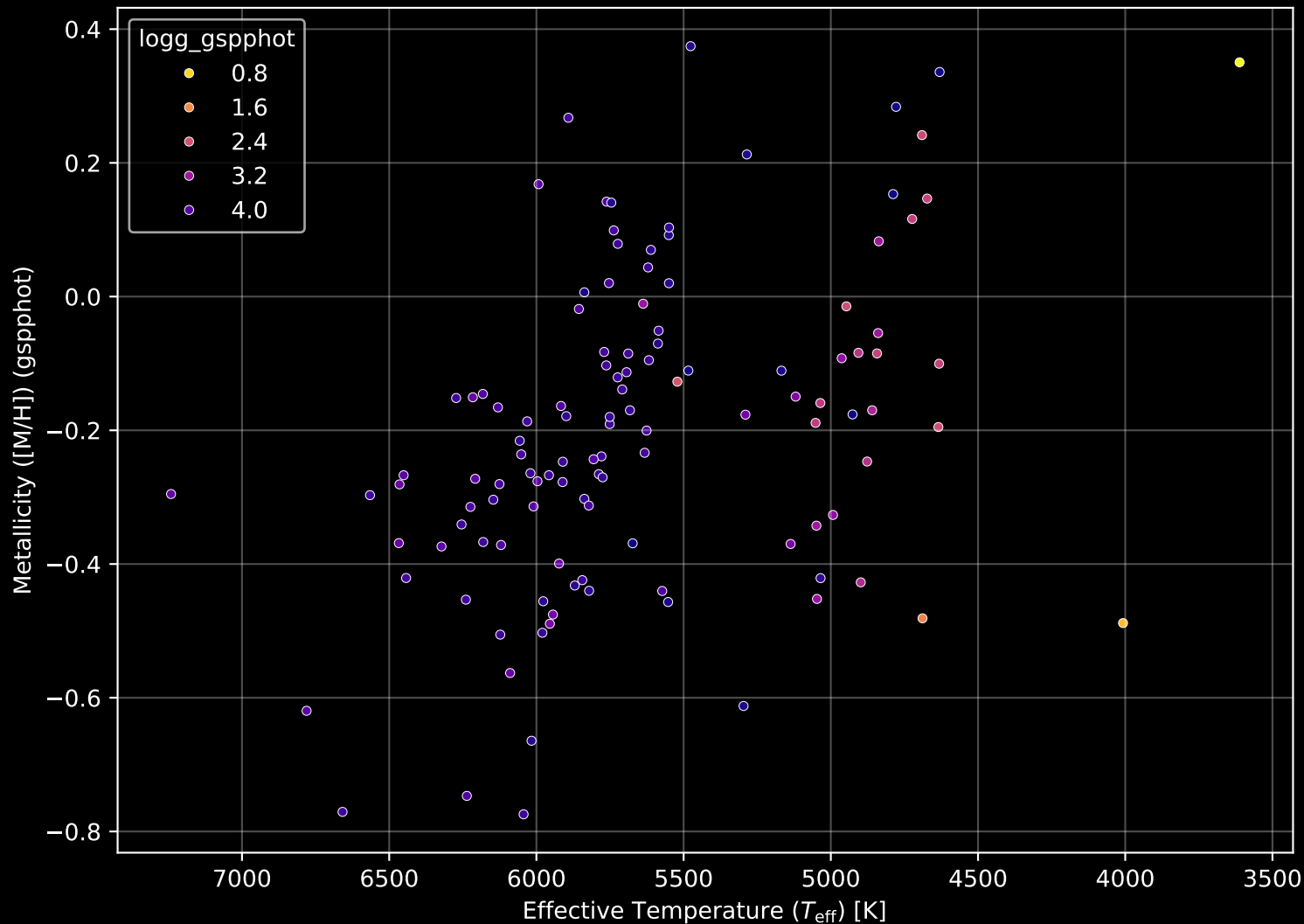
GALAH DR4 Field: [7209] Stellar Population Parameters (n= 119)
